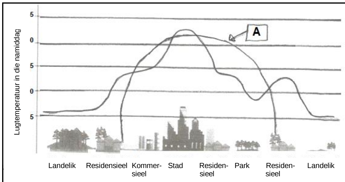
FIGUUR 1.4 STEDELIKE HITTE – EILAND
