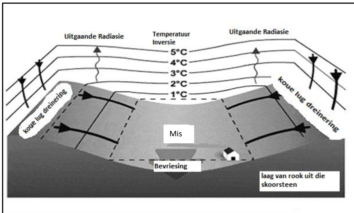
FIGUUR 2.4: KATABATIESE WIND
