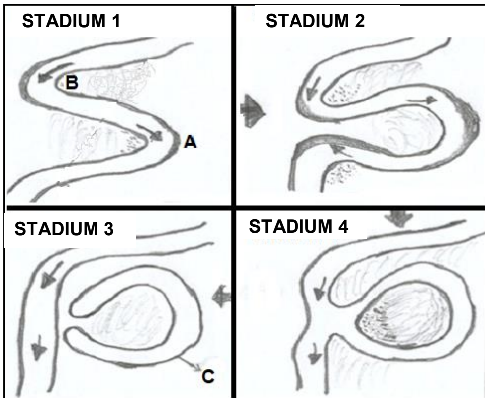
FIGUUR 1.6 KRONKELENDE RIVIER
