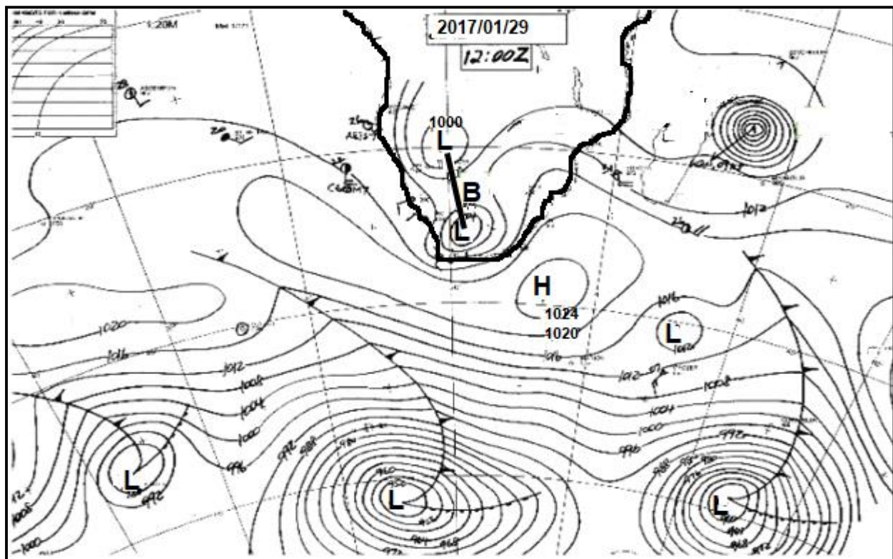
FIGUUR 1.3: SINOPTIESE WEERKAART
