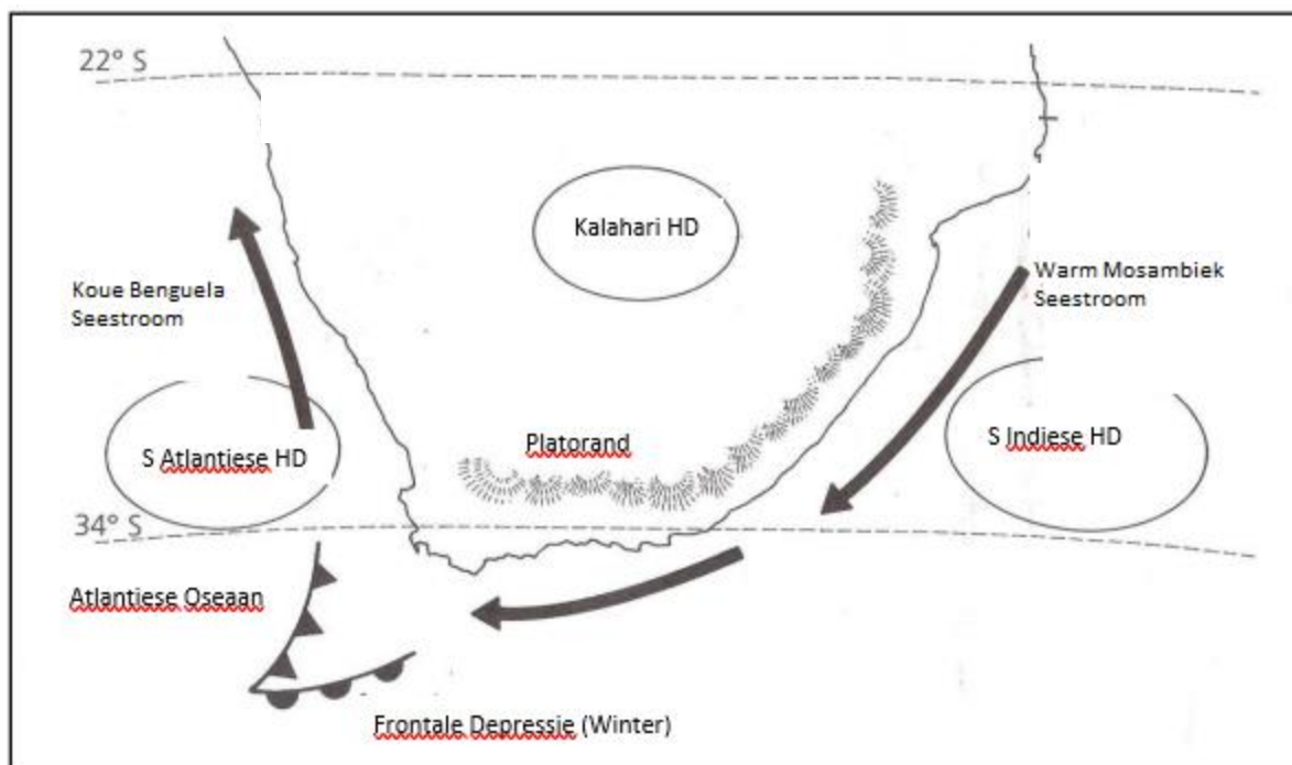
FIGUUR 2.1 FAKTORE WAT SUID-AFRIKA SE WEER BEÏNVLOED
