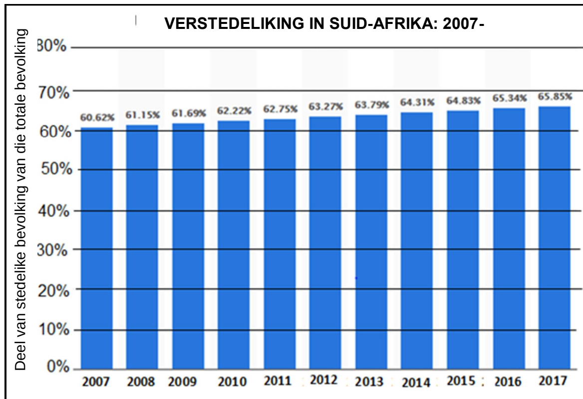
FIGUUR 4.4: VERSTEDELIKING
