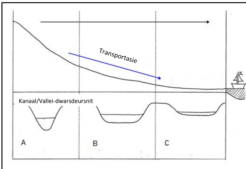
FIGUUR 1.5: 'N DWARSPROFIEL VAN 'N RIVIERKANAAL.
