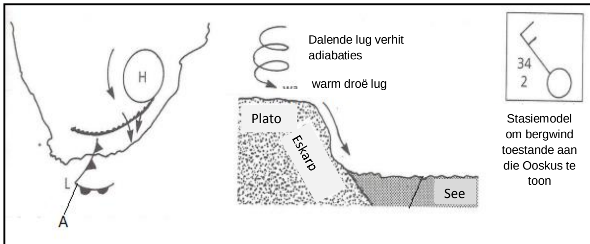
FIGUUR 1.1: BERGWINDTOESTANDE
