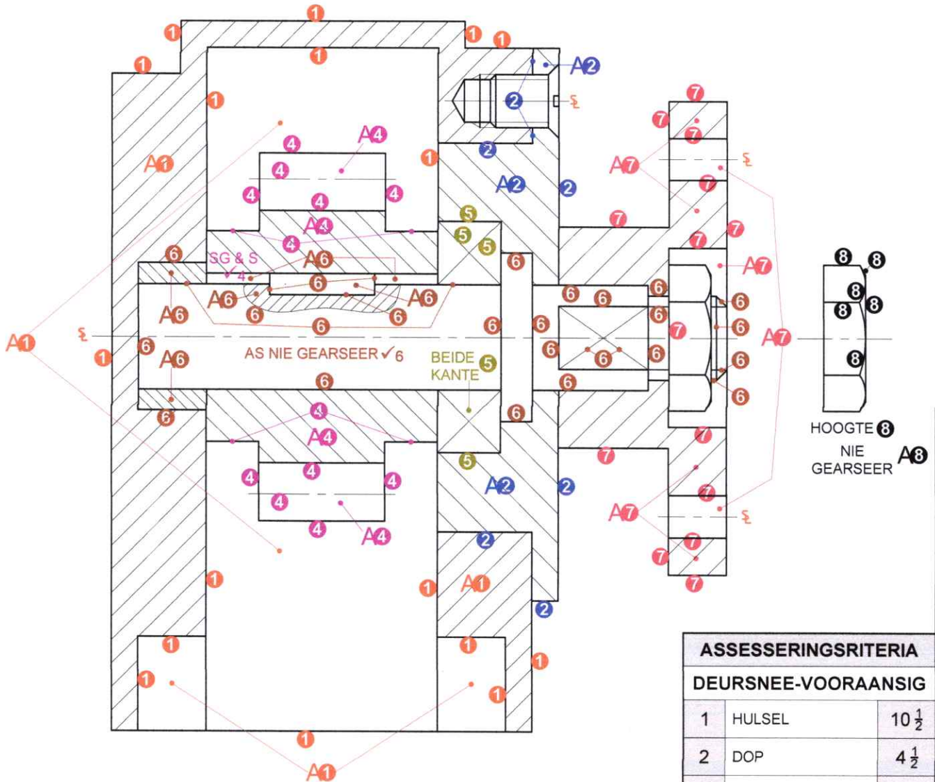
ALTERNATIEVE VERGROTE M10-SKROEF PUNTTOEKENING
