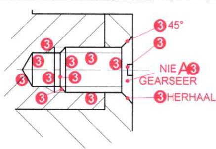
VERGROTE M10-SKROEF PUNTTOEKENING
