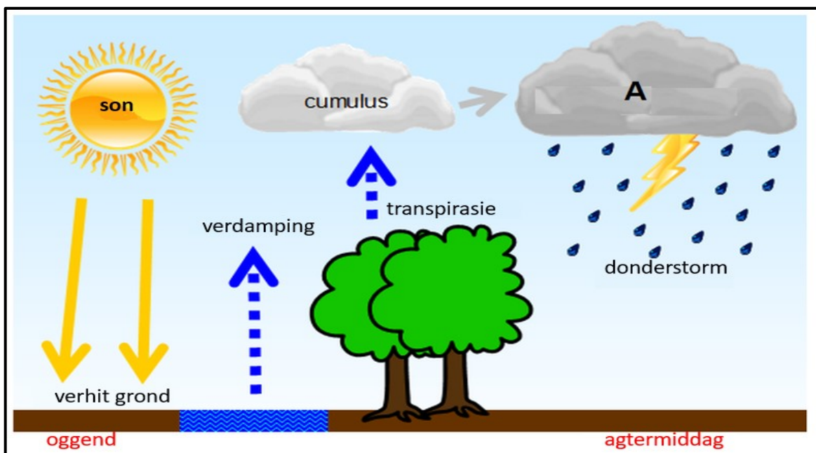
FIGUUR 1.4: KONVEKSIEREËNVAL
